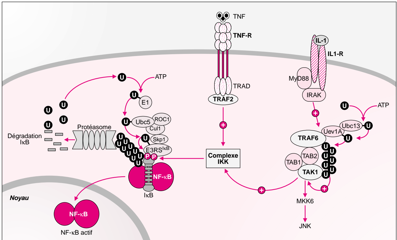
Figure 1. Deux aspects des fonctions de l'ubiquitinylation dans la voie d'activation de NF- \kappa B. Dans la voie de signalisation par le TNF (tumor necrosis factor), l'ubiquitinylation de la sous-unité inhibitrice I \kappa B, induite après activation du complexe IKK (I \kappa B kinases) et phosphorylation de I \kappa B, conduit à la dégradation de l'inhibiteur et à la libération de NF- \kappa B actif. De façon différente et nouvelle, dans la voie de signalisation du récepteur de l'interleukine-1, l'ubiquitinylation de l'adaptateur TRAF6 est cruciale pour la stimulation de la kinase TAK1 qui va mobiliser la voie d'activation de NF- \kappa B ainsi que la voie JNK. D'autres fonctions de l'ubiquitinylation sont discutées dans l'article.
